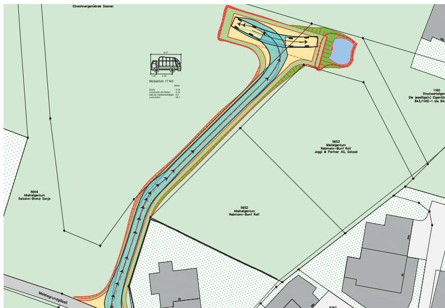
Abb. 5 Schleppkurve, Wendemanöver und die Fahrtrichtung eines Zweiachsers (Kehrtrichtung) (Quelle: Theiler Ing.).
