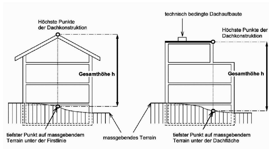
Figur 4.1.a Gesamthöhe
